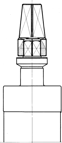
4-kt. Adapter 27/32 mm 6-kt. 19 mm DN 25-80 6-kt. 27 mm DN 100-150 6-Kt. 50 mm DN 200-300
